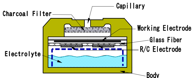
图 2：电化学式气体传感器的构造
